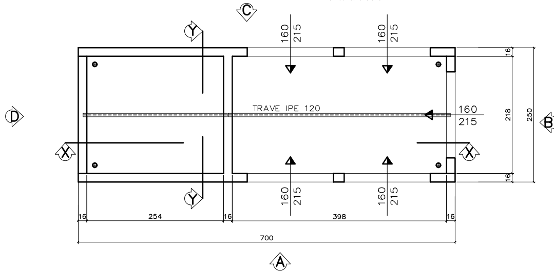
SEZIONE X-X
