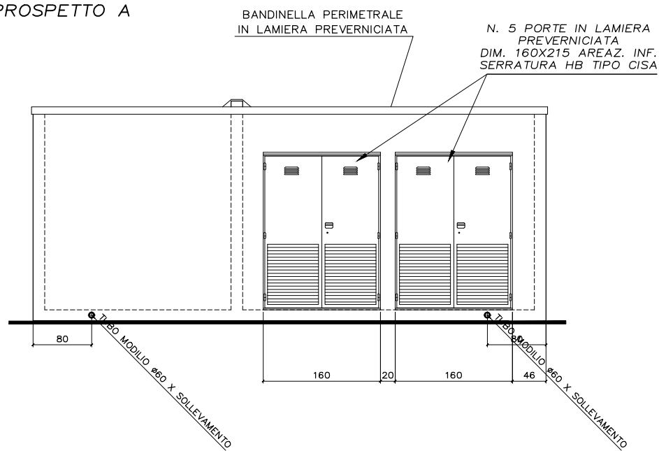
PROSPETTO A
