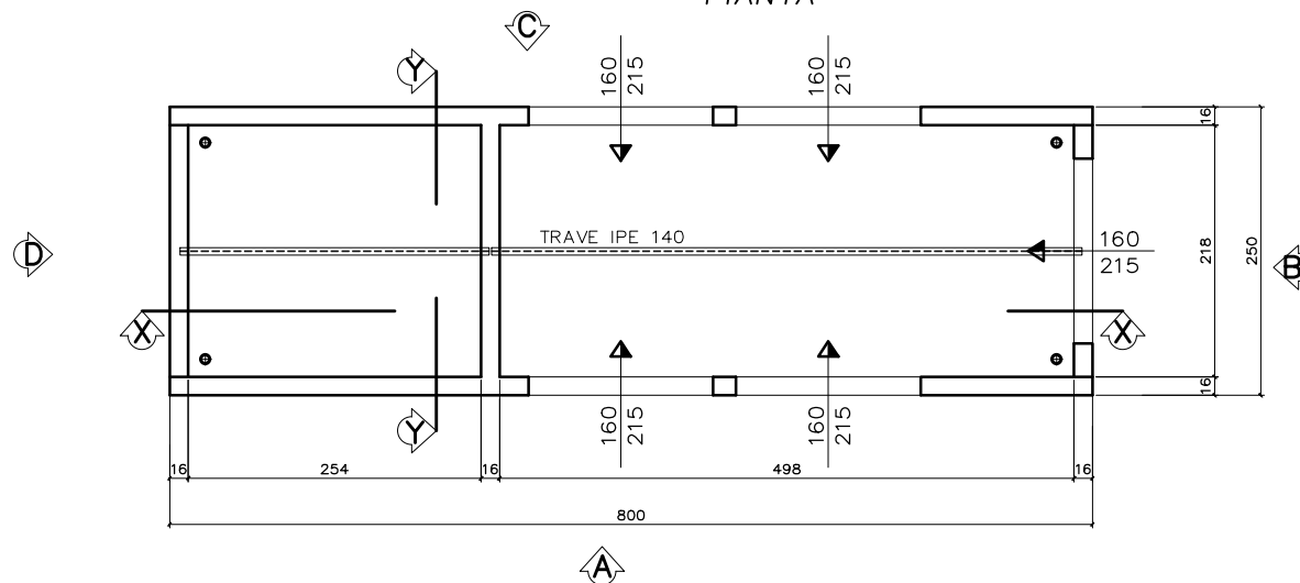
SEZIONE X-X
