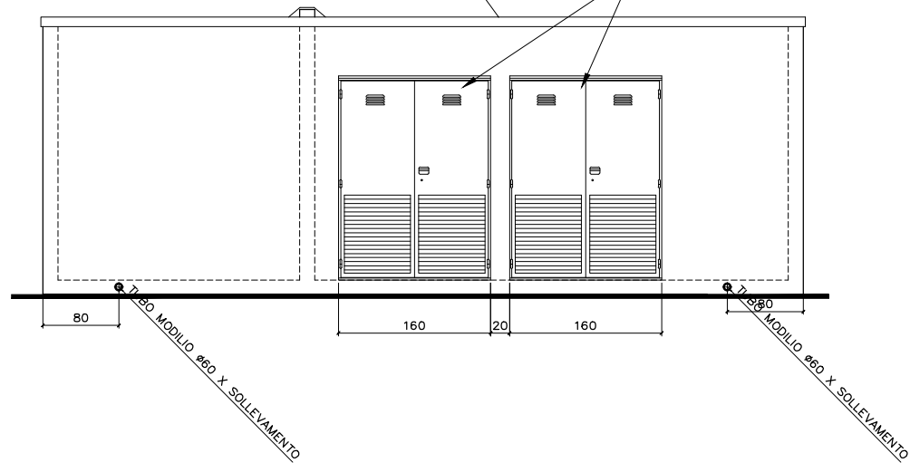
PROSPETTO C
