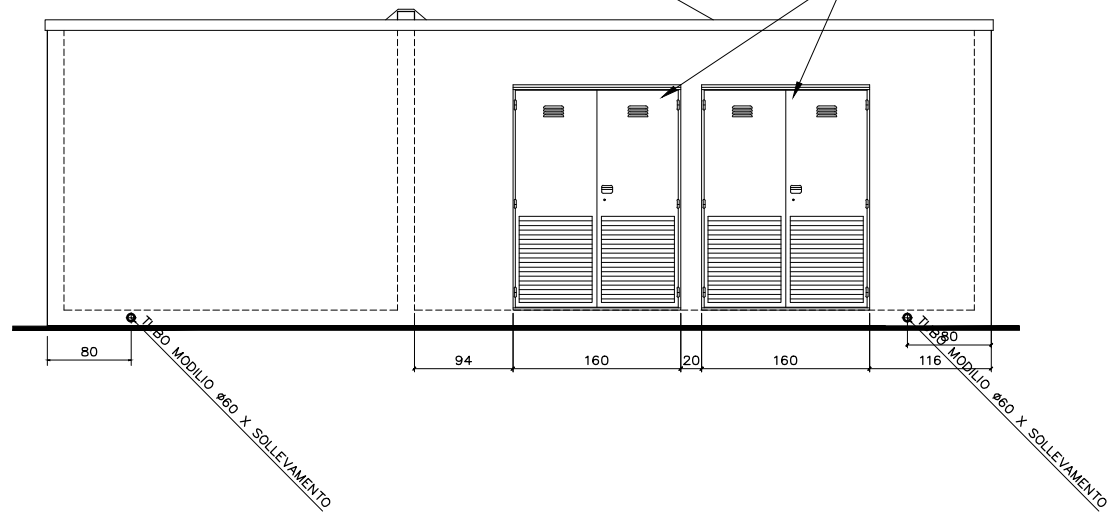
PROSPETTO C
