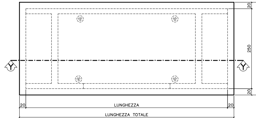
PIANTA PLATEA DI FONDAZIONE
