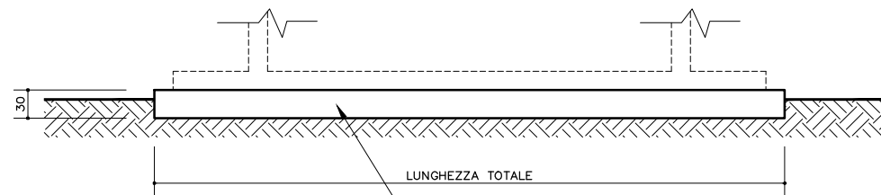
SEZIONE Y-Y
