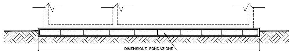
SEZIONE Y-Y
