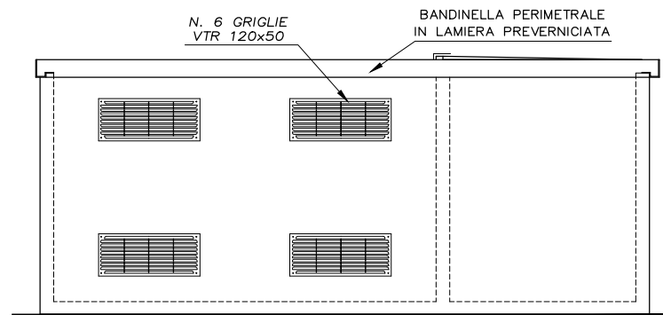
PROSPETTO C
