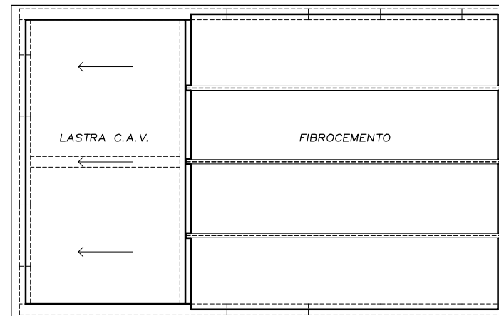
PIANTA COPERTURA SP. 16-20 cm + FIBROCEMENTO
