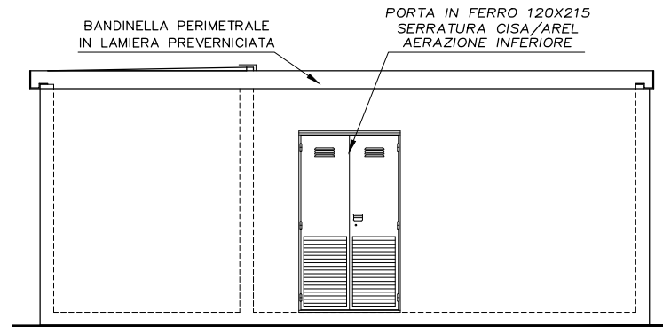
PROSPETTO A
