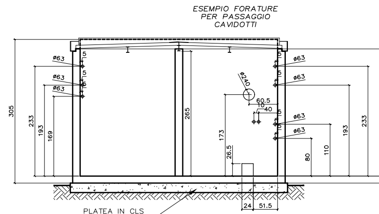
SEZIONE Y-Y
