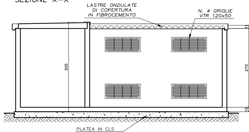
SEZIONE X-X
