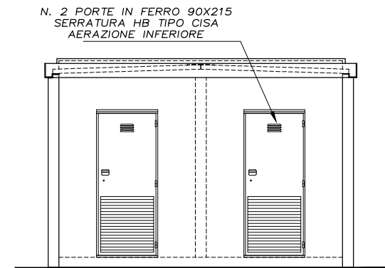
PROSPETTO D
