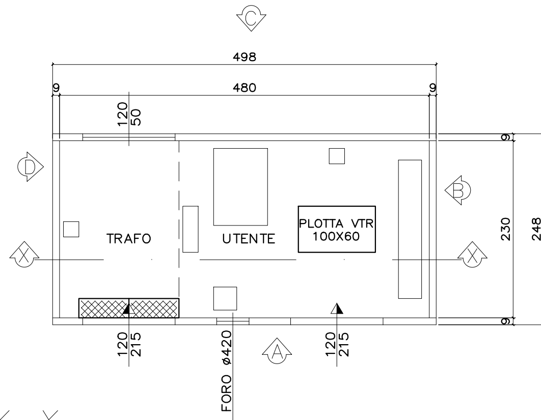
PIANTA
