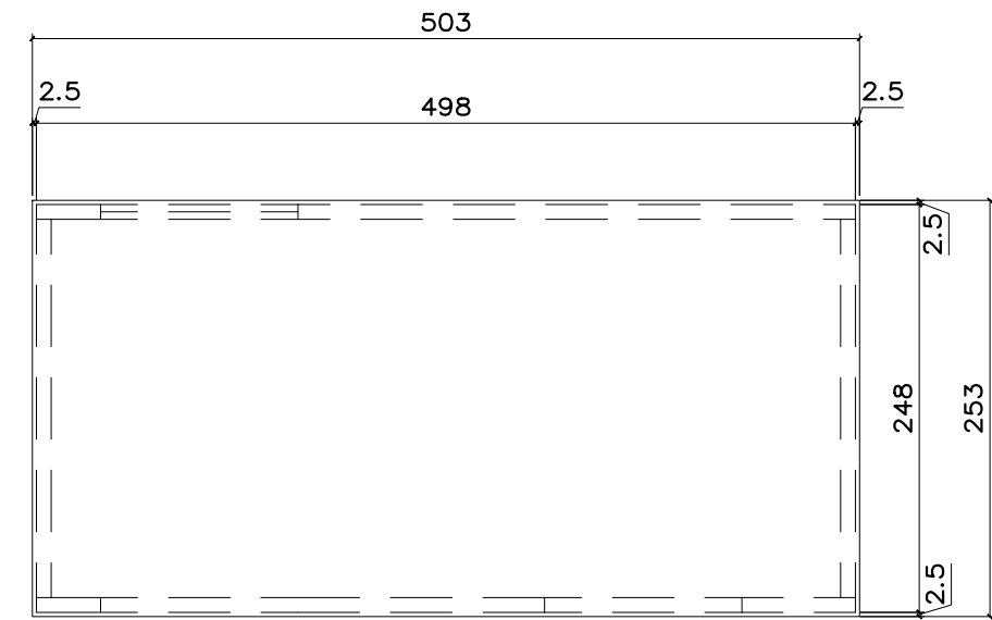
PIANTA COPERTURA SP. CM. 9
