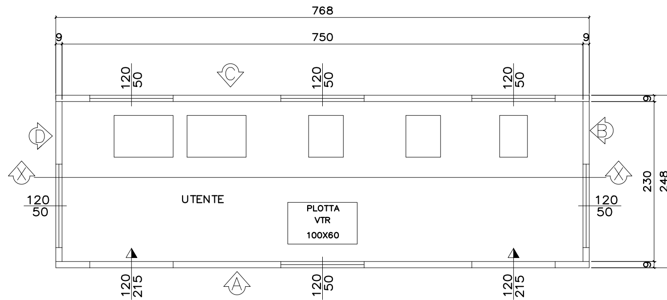
PIANTA
